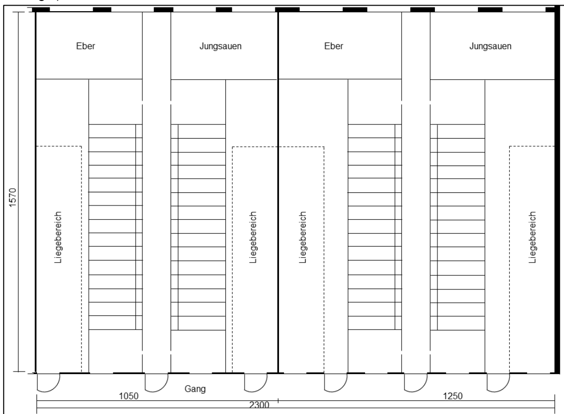
Abbildung 2 Skizze der Deckzentren an der LSZ Boxberg (links: 2 Flächenbucht mit hydraulischen Kippständen; rechts: 3-Flächenbucht mit Selbstfang-Fressliegebuchten)
